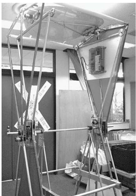
第10回中学生ロボコンで出展されたマシン＝高専で
